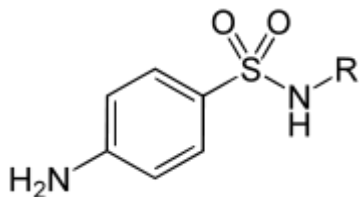
4-аминобензолсульфонамид
